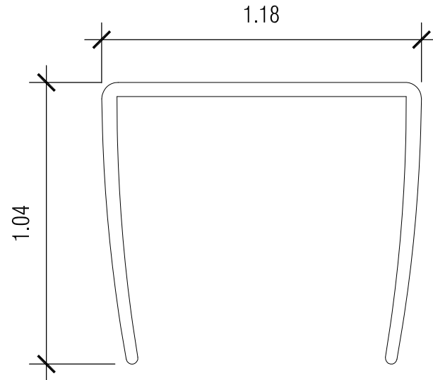
1 SIDE VIEW scale: 2:1
