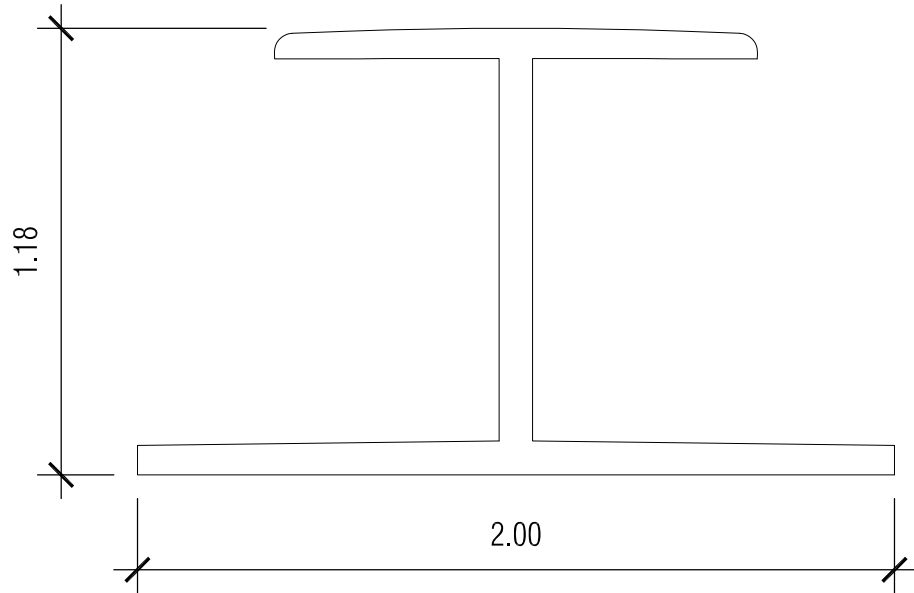
1 SIDE VIEW scale: 2:1
