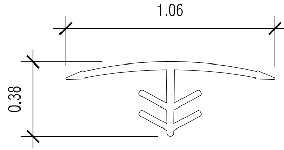
1 SIDE VIEW scale: 2:1
