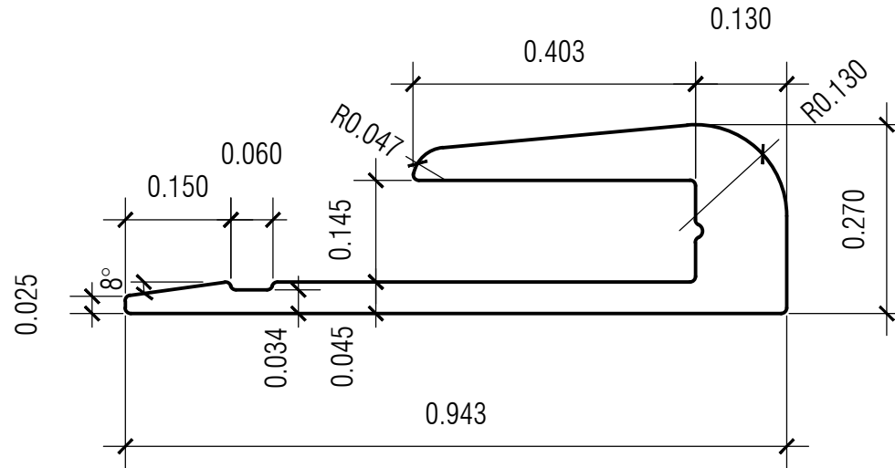
1 SIDE VIEW scale: N T S
